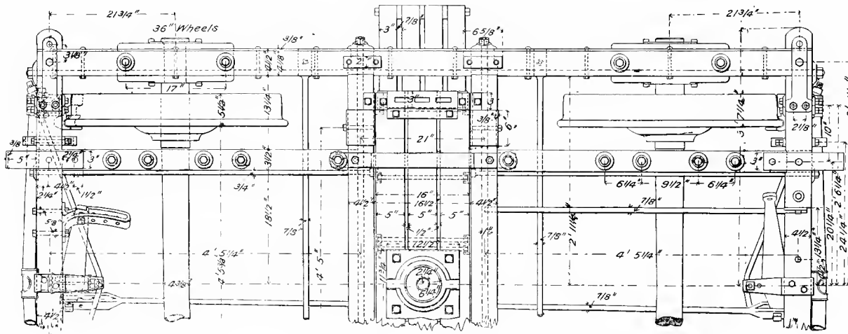
Fig. 4814. Half Plan.
